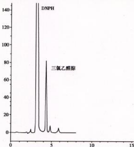
图 1 色谱标准图
